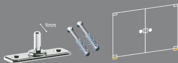
HE 1013A Pivô para dobradiça pino fixo
