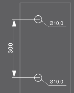
PUXADOR 400 / 500
